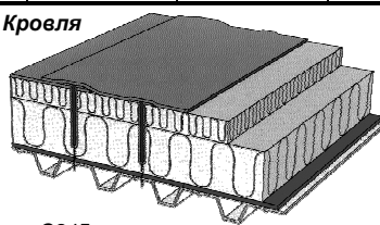
Кровля
